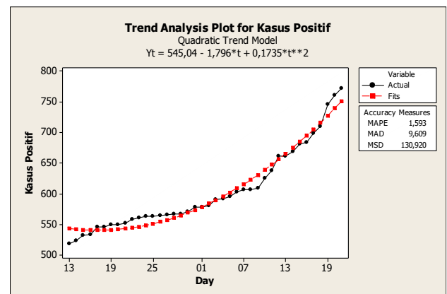
Gambar 4. Uji Trend Kuadratik
