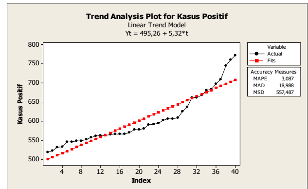
Gambar 3. Analisis Trend Linear
