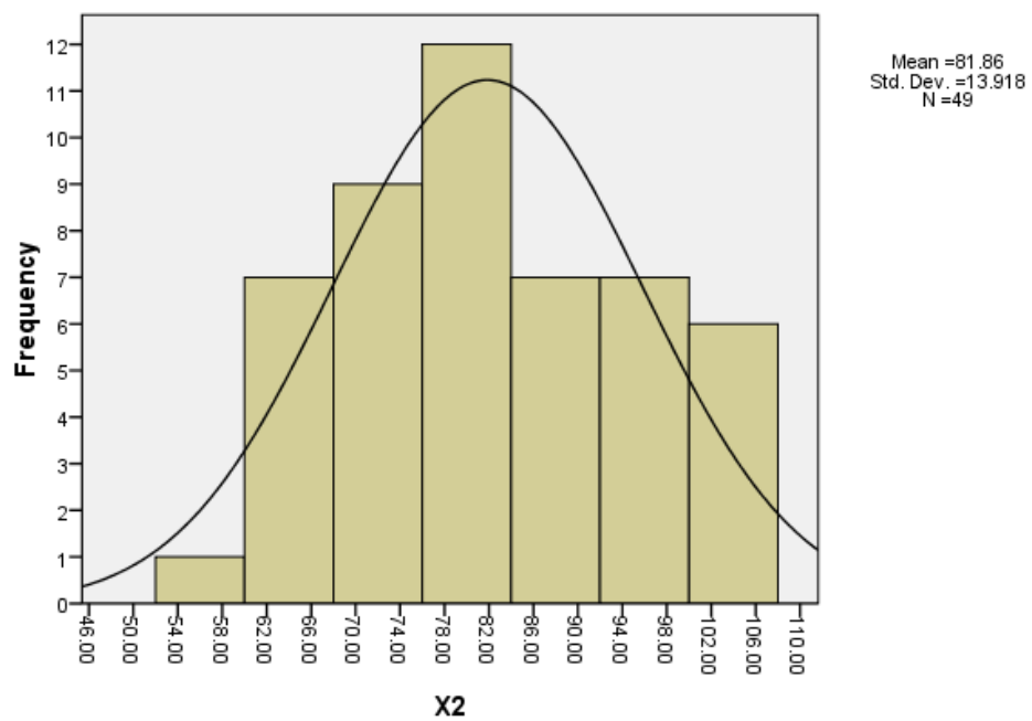
Gambar 3. Kurva Normal Skor Lingkungan Sekolah
