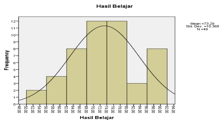
Gambar 4. Kurva Normal Skor Hasil Belajar.
