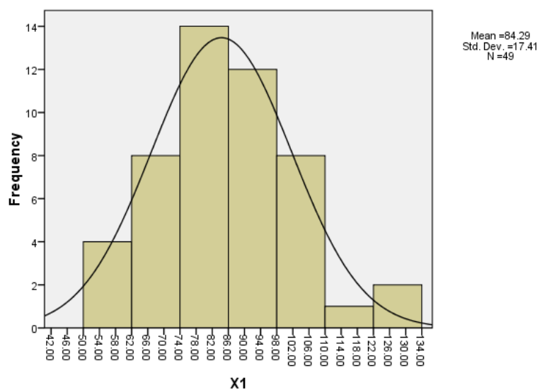
Gambar 2. Kurva Normal Skor Disiplin Belajar
