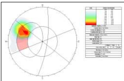
Gambar 8. Analisis Potensi Longsoran Bidang Pada Lereng Berdasarkan Software Dips 6.008
