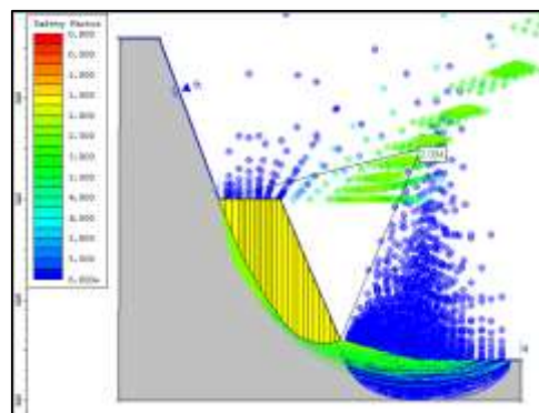
Gambar 15. Nilai Fk Lereng kondisi Jenuh pada bagian bawah
