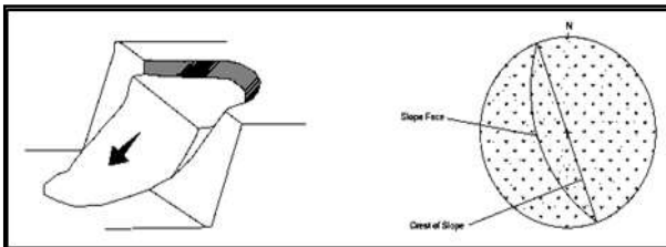
Gambar 5. Geometri Longsoran Busur
