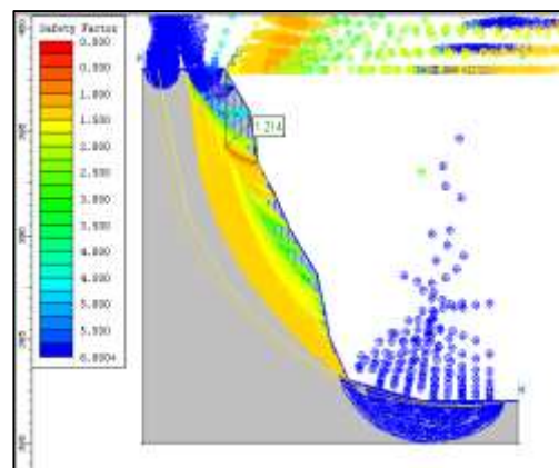
Gambar 10. Nilai FK Lereng Pada Kondisi Jenuh
