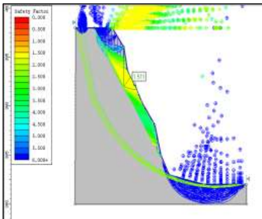
Gambar 12. Nilai FK Lereng Pada Kondisi Kering
