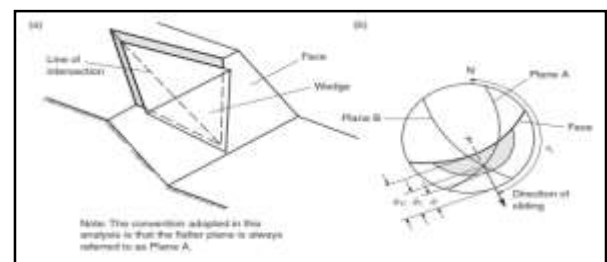
Gambar 3. Geometri Longsoran Baji
