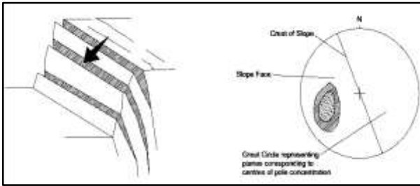
Gambar 4. Geometri Longsoran Guling
