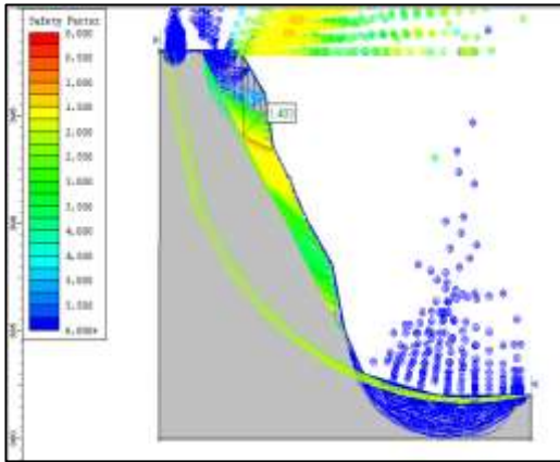
Gambar 11. Nilai FK Lereng Pada Kondisi Asli
