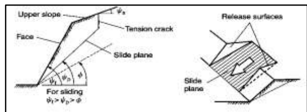
Gambar 2. Geometri Longsoran Bidang
