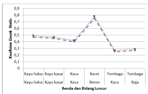
Gambar 16. Grafik Perbandingan Koefisien Gesek Statis Sistem dengan Alat Standar
