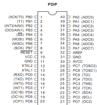
Gambar 5. Konfigurasi Pin ATmega16A [8]
