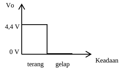
Gambar 12. Hubungan Keadaan Phototransistor dengan Tegangan Keluaran
