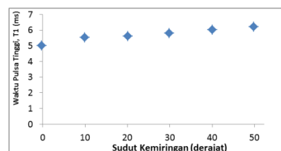
Gambar 14. Grafik Pengaruh Sudut Kemiringan Terhadap Waktu Pulsa Tinggi (T1)
