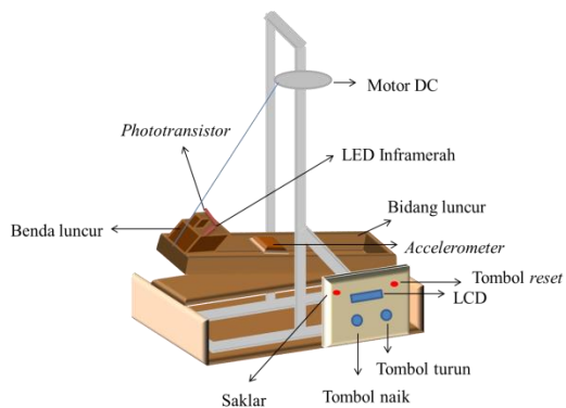
Gambar 8. Ilustrasi Set Eksperimen Penentuan Koefisien Gesek Statis Benda pada Bidang Miring Berbasis Mikrokontroler
