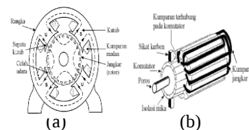
Gambar 1. Konstruksi Motor Arus Searah Bagian Stator (a) dan Rotor (b) [2]
