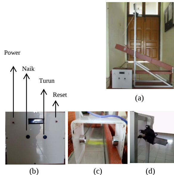
Gambar 10. Foto Hasil Rancangan Sistem: a) Set Eksperimen, b) Panel Depan, c) Sensor Phototransistor dan LED, d) Motor DC
